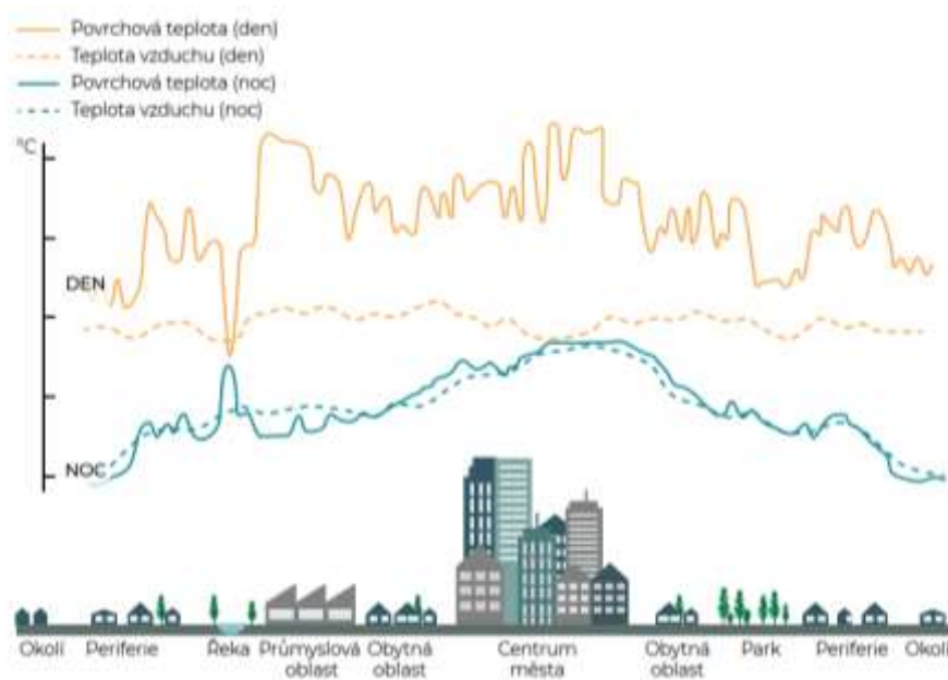
Obrázek 1.3: Průběh teplot během dne a noci
