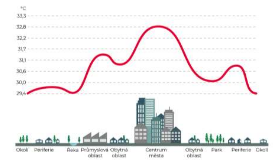
Obrázek 1.2: Schéma tepelného ostrova
